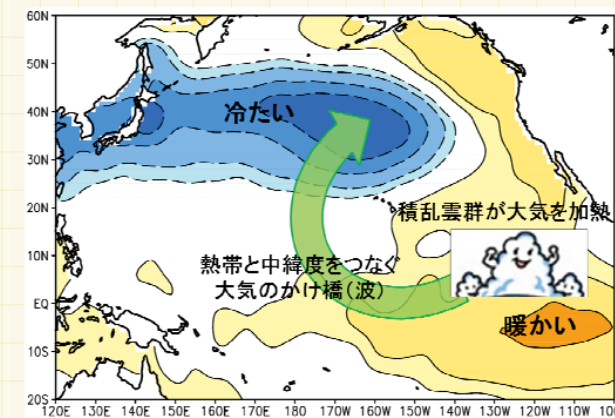
図2: 赤道域の海面水温が「大気のかげ橋」を通じて中緯度の気候・海洋に影響するという説を示した図。
