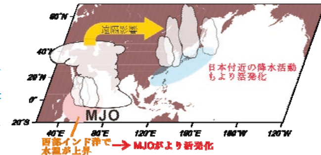
MJOと日本の冬の降水の関係と、地球温暖化の影響の模式図
