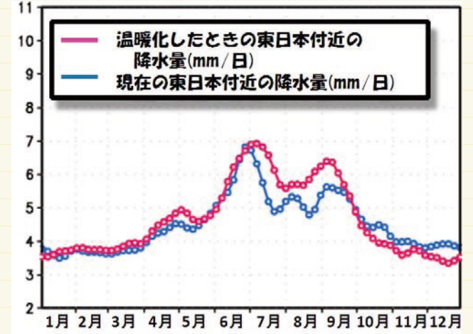
図2：東日本付近の降水量の将来変化
