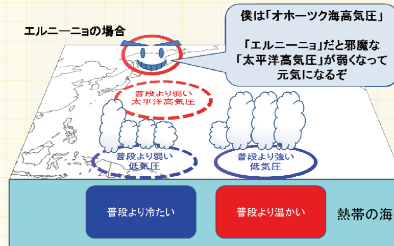
図3: エルニーニョとオホーツク海高気圧の関係を示した説明図。温かい海の上では空気が軽くなって雲や低気圧が生じ、その空気が上空から北に運ばれて北側に高気圧が出来る。エルニーニョが発生すると熱帯太平洋は西の方が普段より冷たくなるため、日本の東の海上の太平洋高気圧は普段より弱くなり、オホーツク海高気圧の影響を受けやすくなる。
