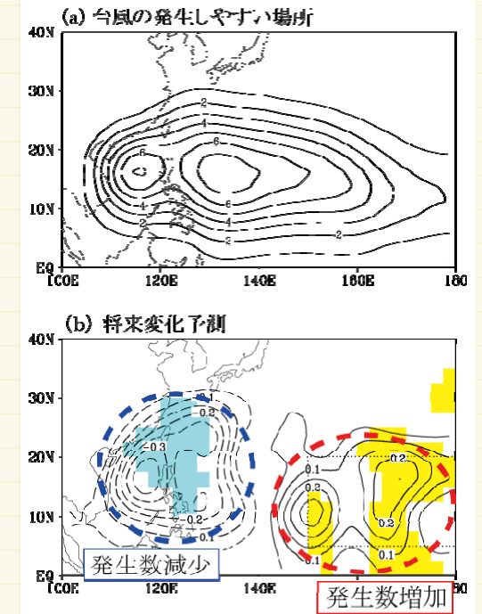
図3：(a) 5つの気候モデルが再現した台風発生数の分布。現実とよく合っている。(b) モデルが予測する、発生数の将来変化(実線は増加、破線は減少)。5つのモデルの予測傾向が一致する地域に色をつけて示してある。
