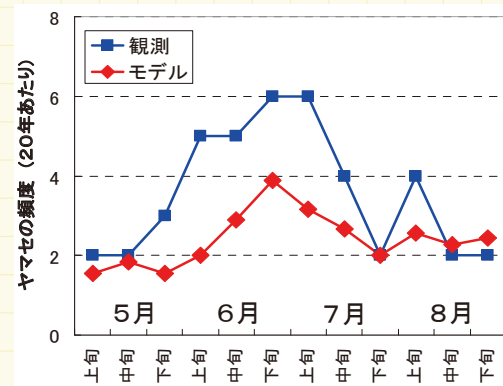
図2: 現在の20年間(1981～2000年)におけるヤマセの発生回数(20年間の合計)。青色線は観測、赤色線は全てのモデルの平均回数を示す。
