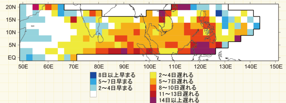
図2：地上付近でモンスーン西風が吹き始める時期（雨季の開始時期）が、温暖化によってどのように変化するかを示したものの。
