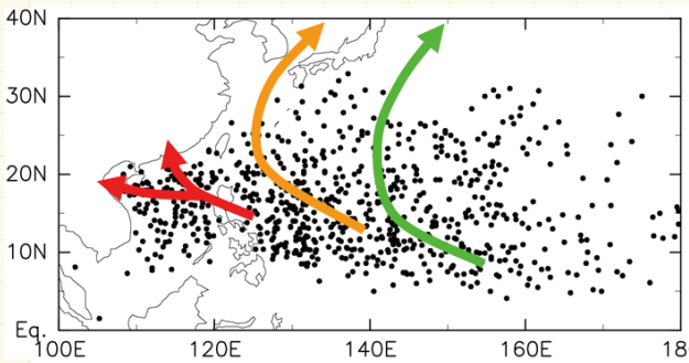
図2：1979-2008年の台風の発生地点(黒点)と発生場所ごとの台風の取りやすい経路(矢印)
