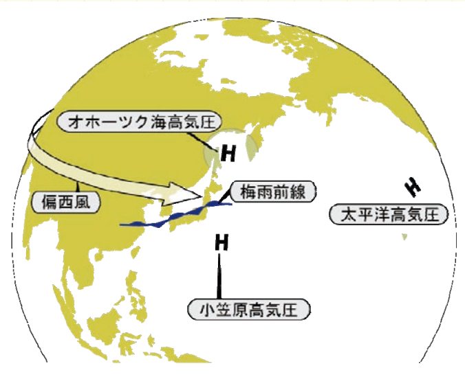
図1：7月頃の梅雨前線と高気圧、偏西風の様子（出典：現代用語の基礎知識）。
