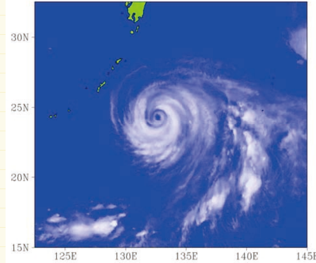
図1：台風の衛星画像
