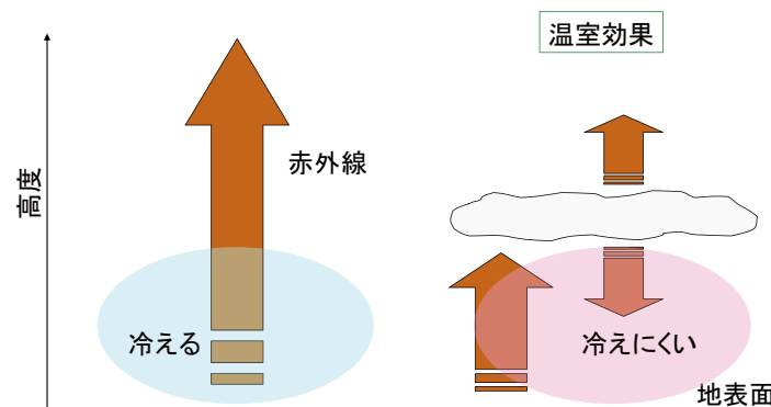
図2：雲による温室効果の概念図
