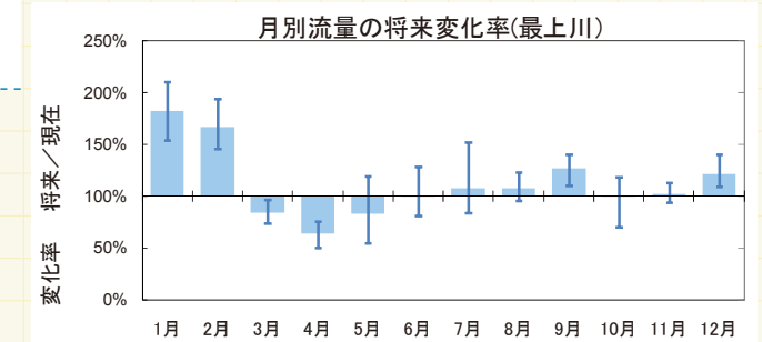
図3：最上川の月別流量の将来変化。棒グラフはCMIP3マルチモデルの平均を示し、I型の線は予測結果のばらつきを表す。
