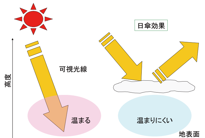
図1：雲による日傘効果の概念図
