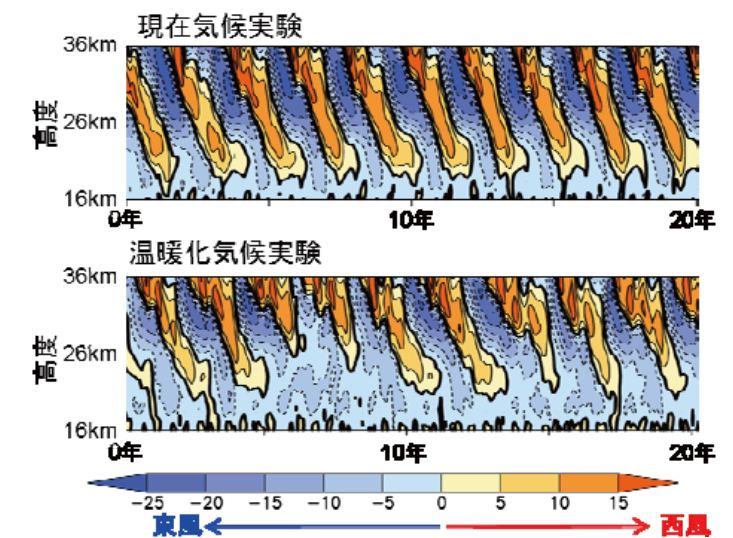
赤道に沿って平均した東西風(シミュレーション結果)。西風域と東風域が時間とともに上から下へと伝播しつつ交代するQBOの特徴が再現されている。
