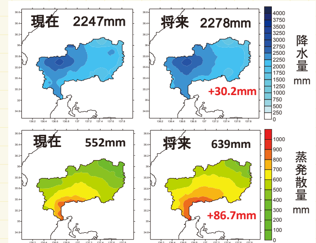
図2：木曾川流域における現在(左：1979-2003)と将来(右：2075-2099)の年間降水量(上)と年間蒸発散量(下)の変化。
