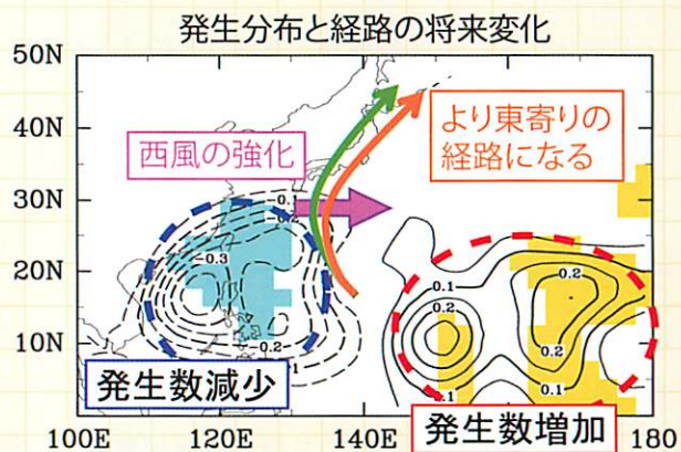
図2：台風の発生分布と、日本付近での経路の将来変化の模式図。発生分布の変化は等値線で表わされ、モデルの予測傾向が一致する地域に黄・水色をつけて示してある。発生分布は5種類のCMIP3モデル、経路変化はそれらに加え2種類のより台風の表現にすぐれた気象庁気象研究所20km格子高解像度大気モデルの将来予測結果に基づく。
