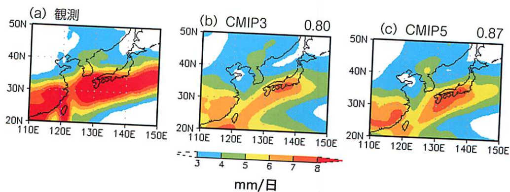
図: 6月の日本付近の雨量分布 (mm/日)。1981-2000年の平均。(a) 観測値、(b) CMIP3モデル、(c) CMIP5モデル。(b) と (c) の外側の右上にある数字は観測値にどの程度似ているかを表す数値 (相関係数) で、1に近いほど類似。
