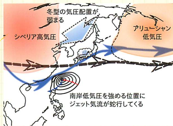
図1：温暖化した21世紀末での冬の模式図。長い矢印はジェット気流の位置、等値線は気圧配置。各々、破線が現在、色が将来。
