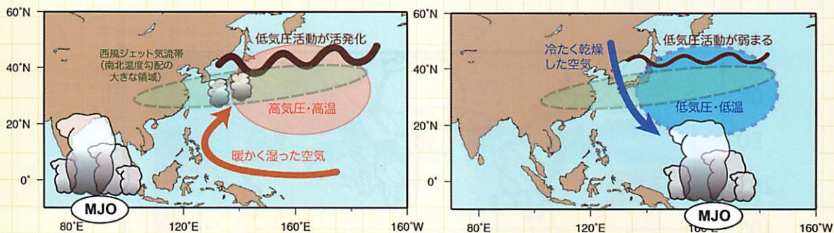
図2：現在の冬季 MJO と MJO による亜熱帯・中緯度への影響の模式図。MJO が（左）東部熱帯インド洋で、（右）西部～中部熱帯太平洋域で発達している場合。
