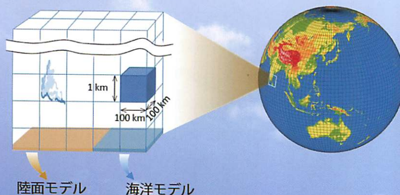
大気モデルの格子イメージ
