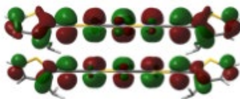
図2 PTNT2T のモデル化合物の結晶構造：（上）真上から見た構造、（下）真横から見た構造に分子軌道を重ね合わせた。TNT 骨格同士が大きく重なり合う core-to-core スタッキングが形成されている。このスタッキング構造により、分子軌道の重なりが通常の3倍となり、分子間でも効率的に電荷を輸送できる。
